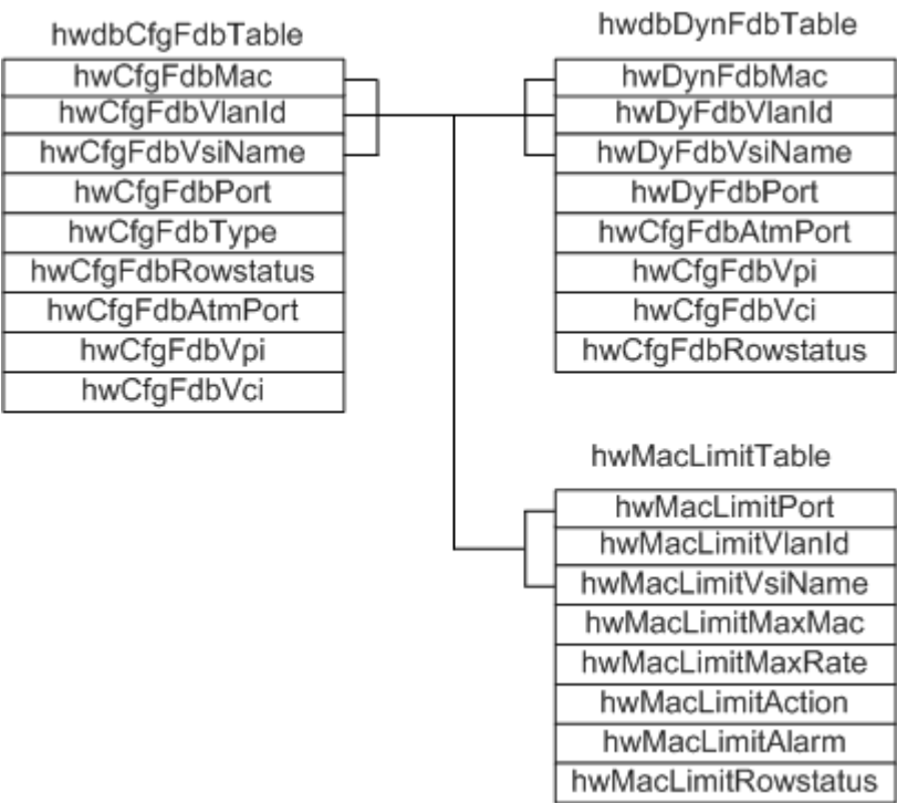
图 70-1 静态 MAC 地址表 hwdbCfgFdbTable 、动态 MAC 地址表 hwdbDynFdbTable 以及 MAC 地址学习限制表 hwMacLimitTable 的表间关系图
